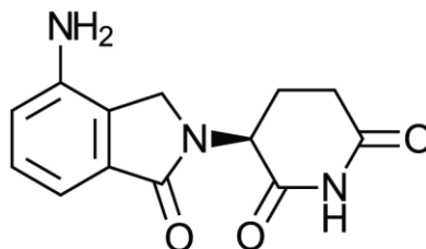
Lenalidomide
