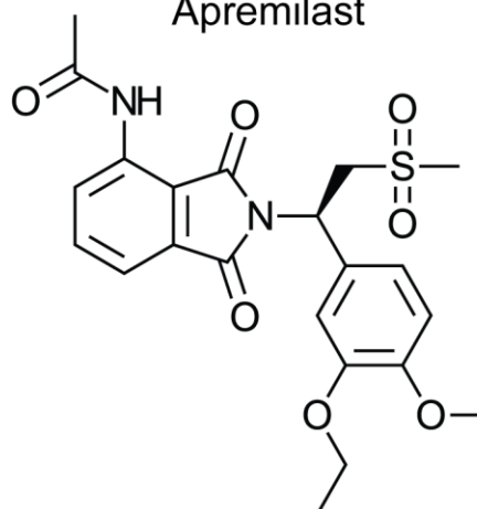
Apremilast
