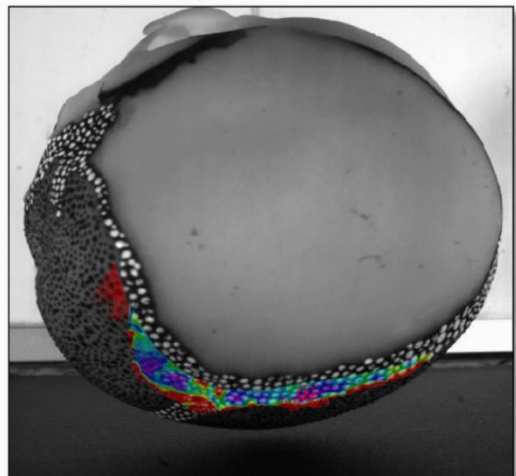
(f) Vertex impact test
