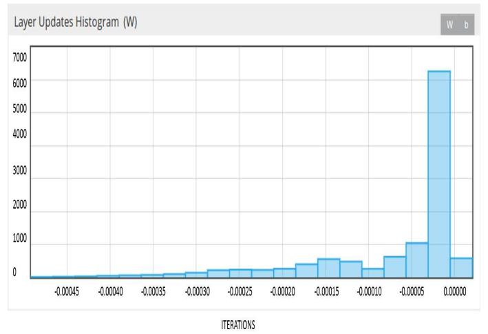
Fig. 12: Histogram of Layer Updates
