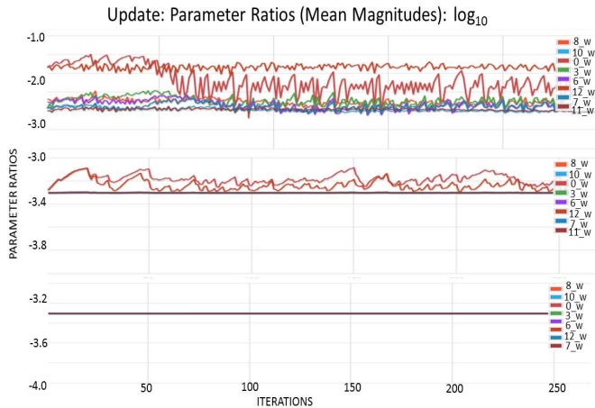
Fig. 7: Parameter Ratios
