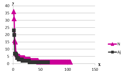
Рис. 6. Залежність Есту-Зіпфа (3).
