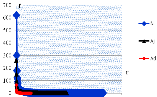
Рис. 4. Залежність Есту-Зіпфа 1.
