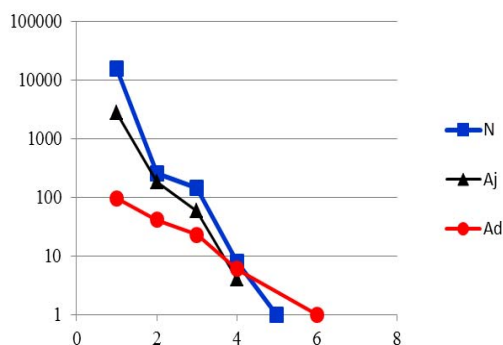
Рис.5. Залежність Есту-Зіпфа 2.
