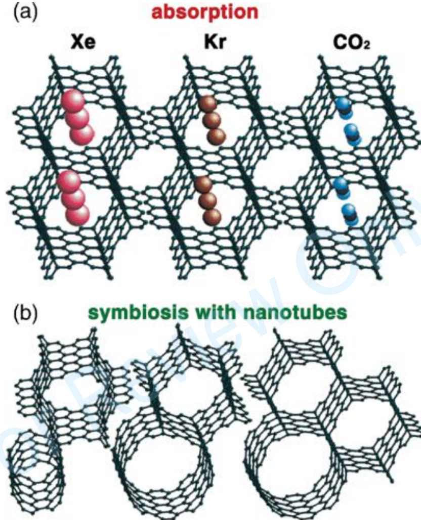
图 26 (a) 蜂窝碳吸收不同气体的能力 (b) 蜂窝结构与碳纳米管共生的独特现象 [122]
