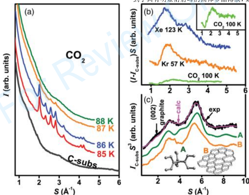
图 25 (a) 凝聚态 CO 2 的电子衍射强度和散射波矢量的关系 (b) 去除碳基底电子衍射的作用后, Kr、Xe 和 CO 2 三种电子衍射强度与散射波矢量的关系 (c) 实验得到的电子衍射强度与计算得到的相比较 [122]
