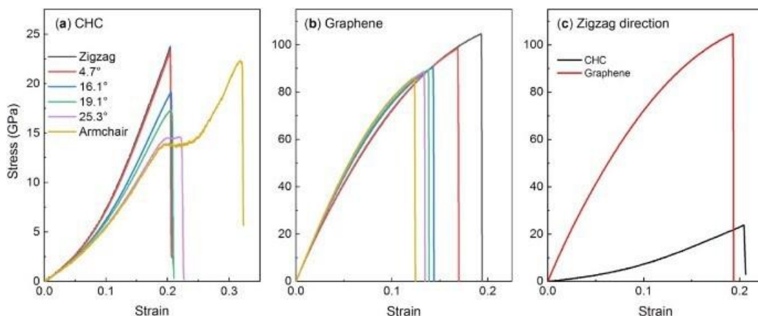
图 17 力学性能对 x-y 平面不同拉伸方向的依赖关系 (a) 蜂窝碳的工程应力-应变曲线 (b) 石墨烯的工程应力-应变曲线 (c) 蜂窝碳和石墨烯在 \theta 为 0^\circ 时的应力-应变关系 [105]
