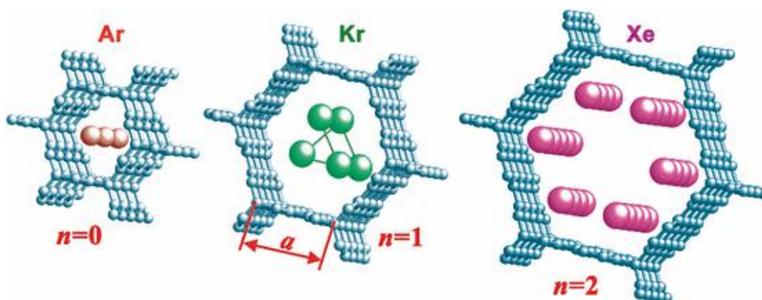
图 27 生长的蜂窝碳晶胞中吸收的 Ar、Kr 和 Xe 原子的最合理排列（氩原子能够插入到 n=0 时的蜂窝结构中，对于较大的氪和氙原子则需要更高 n 值的通道来存放） [41]
