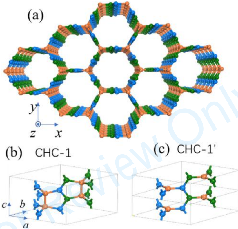
图 9 蜂窝碳 (a) CHC-1 的顶部透视图, 其中的碳原子形成三维蜂窝 (b) CHC-1 的原始晶胞, 绿色的 C1 和蓝色的 C1 原子相对于 c 轴位于不同的平面上 (c) CHC-1 的另一种结构, 其中的 C2 已经解除了二聚体状态 [68]
