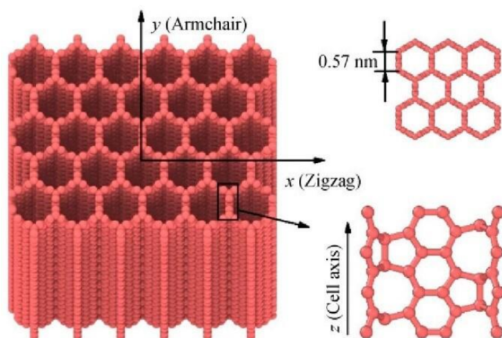
图 7 蜂窝碳结构示意图 [62]
