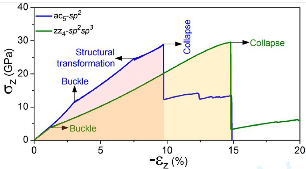
图 22 蜂窝晶格尺寸分别为 l = 9.8 \text{ \AA} 和 l = 10 \text{ \AA} 的两种蜂窝结构的典型应力-应变曲线。(标出了临界变形点和破坏点) 图经文献出版单位许可从文献【53】转载。
