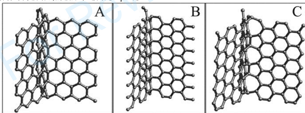
图 8 石墨烯薄膜交叉碰撞产生的三维碳结构 (A) 扶手椅型结构 (B) 锯齿型结构 ( sp^3 构型中四个键原子结线, 不具有六角对称性) (C) 锯齿型结构 ( sp^3 构型中四个键沿着一个结线取向, 具有六角对称性, 位于连接壁中的三键夹角为 120^\circ ) [52]
