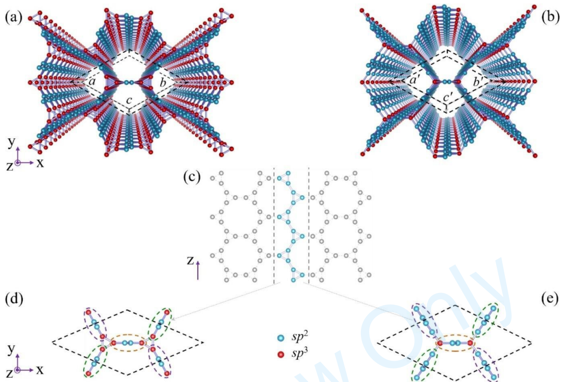
图 12 (a, b) 分别为 KGN-1 和 KGN-2 的俯视图 (虚线框内表示其原始单胞结构, a, b, c 和 a', b', c' 分别为其晶格常数) (c) Kagome 石墨烯纳米片 (浅蓝色部位表示其较薄区域) (d, e) 分别为 KGN-1 和 KGN-2 单胞结构俯视图 (蓝色原子表示 sp^2 杂化, 红色原子表示 sp^3 杂化) [75]
