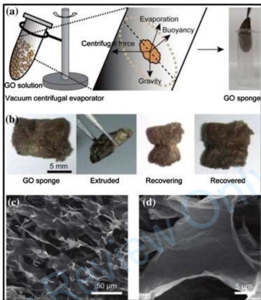
图 32 (a) 三维氧化石墨烯海绵的一种合成方案 (b) 氧化石墨烯海绵的柔韧性测试 (c) 氧化石墨烯表面低倍 SEM 图像 (d) 氧化石墨烯海绵内部高倍 SEM 图像 [144]
