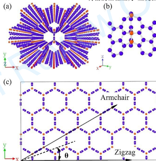
图 16 蜂窝碳结构示意图 (a) 透视图 (b) 结区局域原子结构 (c) 在 x-y 平面内沿不同方向加载的蜂窝碳示意图 [104] 图经文献出版单位许可从文献【104】转载。
