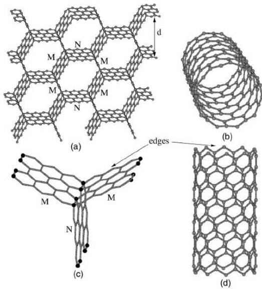
图 2 (a) (3,3) 型的锯齿型碳泡沫结构 (c) 锯齿型碳泡沫连接处结构 (b, d) 与其相对应的锯齿型碳纳米管结构及连接情况 [32]
