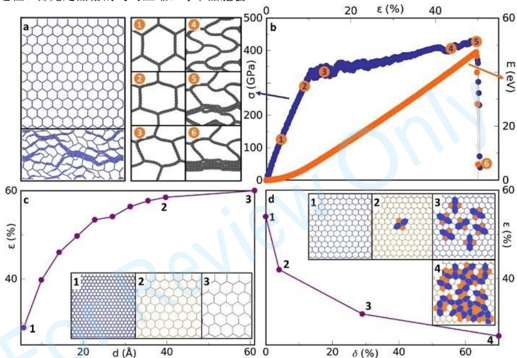
图 15 蜂窝碳的压缩特性 (a) 蜂窝晶格的局部塌陷和蜂窝晶格压缩过程的放大 (b) 蜂窝结构在压缩过程中的应力-应变曲线和能量-应变曲线 (对应于 (a) 中的各个步骤) (c) 破坏应变与晶格尺寸的关系 (d) 破坏应变与缺陷密度的关系 [51]
