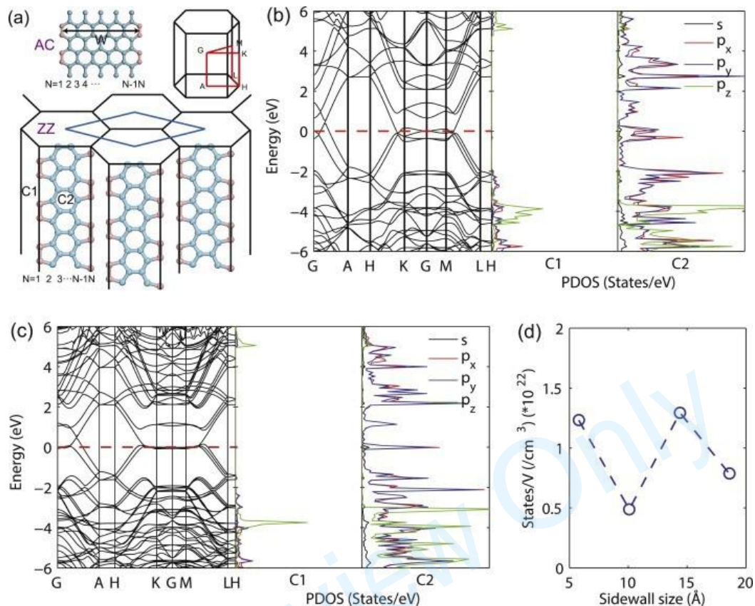
图 11 不同尺寸锯齿型蜂窝碳的电子能带结构。(a) 锯齿型和扶手椅型蜂窝碳侧壁的原子结构, 右上角是第一个用来表示电子结构的布里渊区 (b, c) 不同侧壁宽度的锯齿型蜂窝碳对应的原子能带结构及其态密度投影 (b:5.8 Å;c:10.1 Å) (d) 体积中的费米能级平均值与侧壁尺寸的函数关系 [69]
