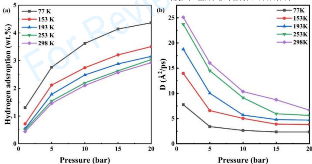
图 28 (a) 氢吸附的等温线 (b) 氢的扩散系数 (分别在 77K、153K、193K、253K 和 298K 条件下测得) [125]
