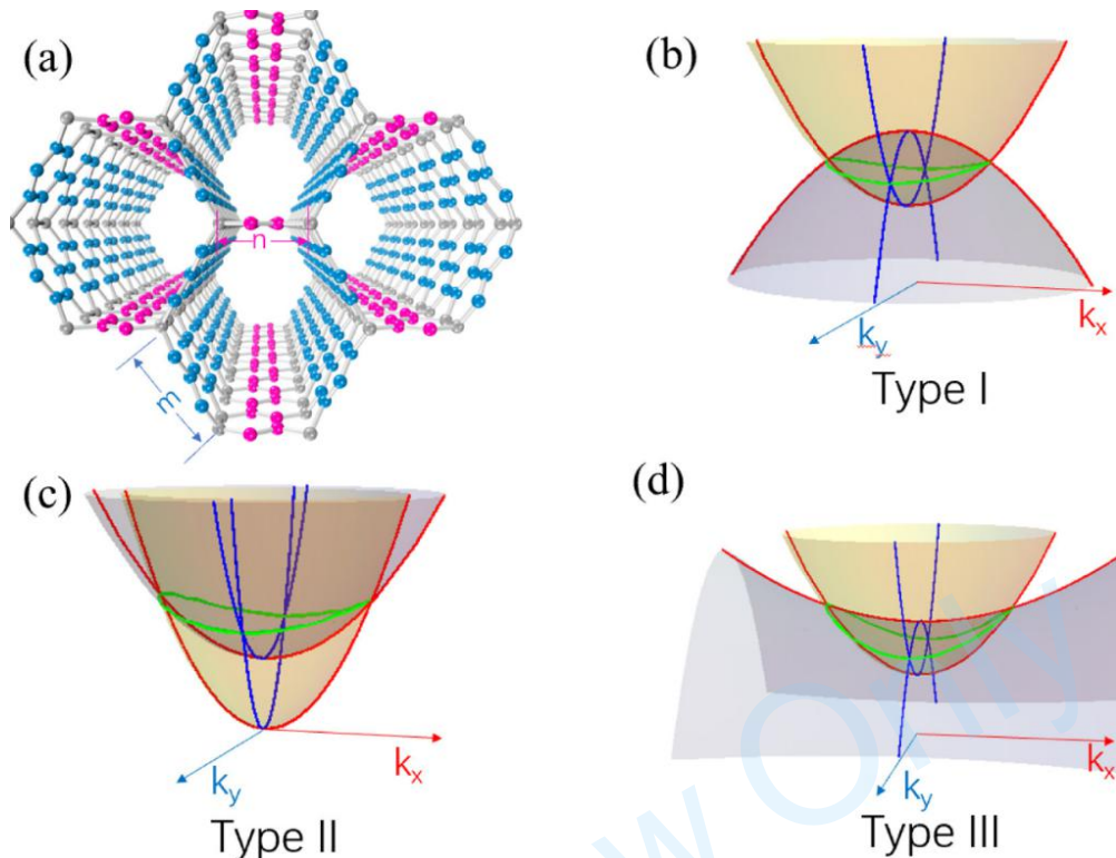
图 10 (a) 由扶手椅形石墨烯纳米带连接形成的碳网络原子结构, 命名为 AGNW- (m, n) (b-d) 由 AGNW- (3, 2) 和 (1, 2) 根据第一性原理计算得到的三种不同类型节点环的特征能量色散图 [68]
