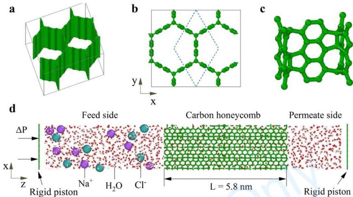
图 29 模拟盒子与海水淡化性能 (a) 任意角度放置的蜂窝碳 (b) 蜂窝碳的垂直视图 (c) 蜂窝碳壁与连接处的原子结构 (d) 模拟盒子示意图 (含有蜂窝碳、水分子、钠离子、氯离子和两片石墨烯片) [131]
