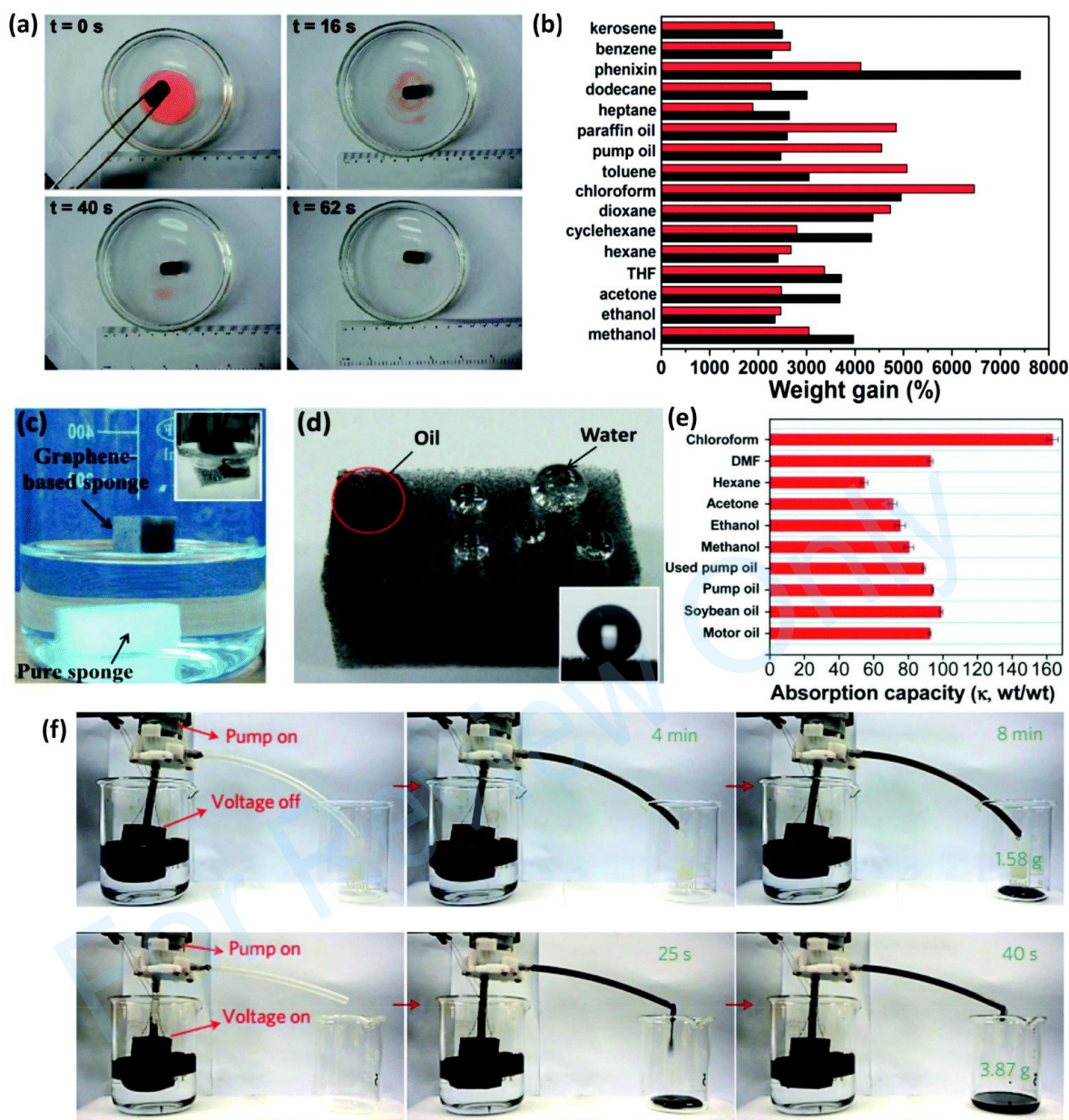
图 33 石墨烯/PVDF 气凝胶 (a) 吸附过程 (b) 吸附容量 (c) 白色海绵和黑色石墨烯基海绵放到水中的图片 (d) 石墨烯基海绵表面的准球形水滴和机油痕迹 (e) 海绵的吸附能力 (f) 焦耳加热的石墨烯基海绵在 0 和 17 V 电压下通过抽吸连续收集海水表面的粘性原油 [166]
