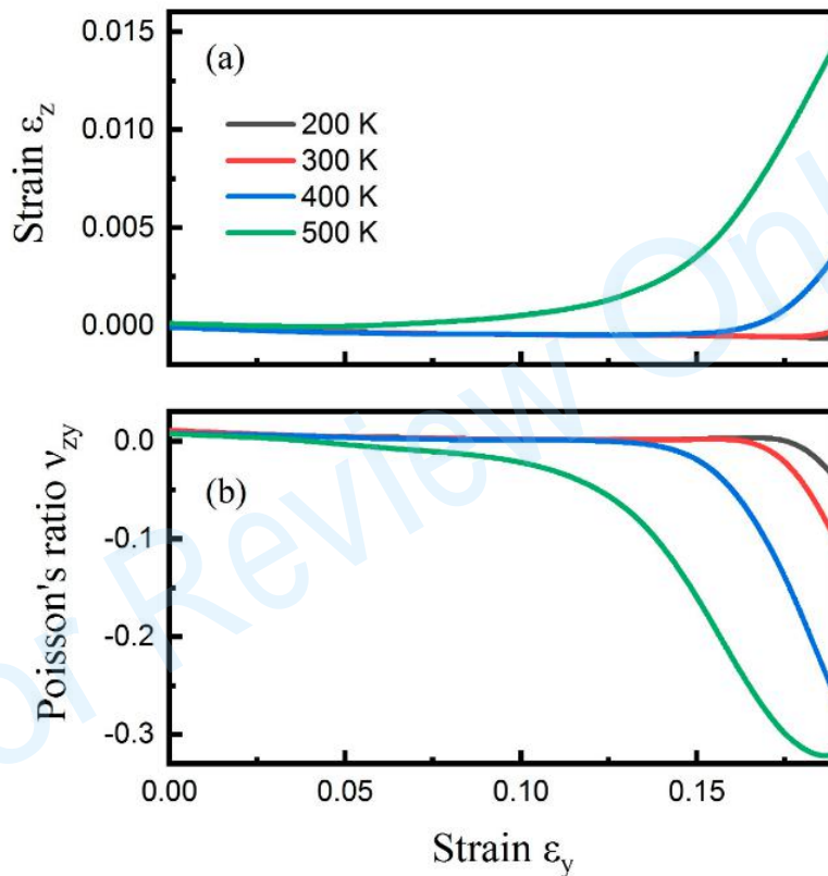
图 19 温度对蜂窝碳在扶手椅方向上单轴拉伸试验中正负泊松比转变的影响 (a) 在 200~500K 的环境下, 测得的工程应力-应变曲线 (b) 不同温度下蜂窝碳对应的泊松比 [107]
