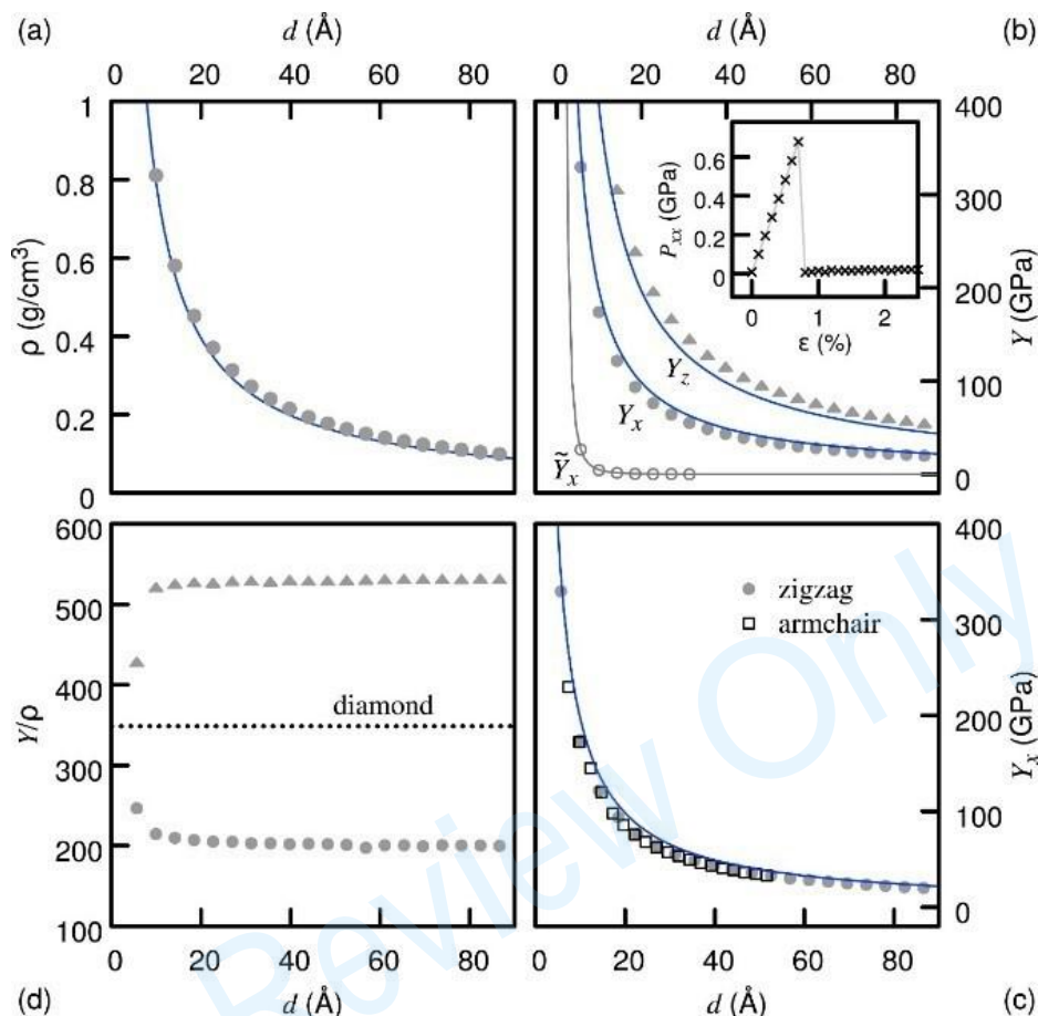
图 13 蜂窝碳的弹性性质 (a) 蜂窝晶格密度与晶格尺寸的关系 (b) 蜂窝杨氏模量与晶格尺寸的关系 (计算值与分析模拟的比较) (c) 两种结构的蜂窝碳在 xy 平面内的杨氏模量与晶格尺寸的关系 (d) 蜂窝杨氏模量与钻石杨氏模量的比较 [51] 图经文献出版单位许可从文献【51】转载。
