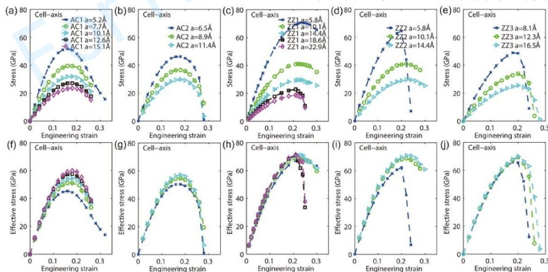
图 18 (a-e) 不同侧壁宽度蜂窝碳在单元轴向拉伸时的应力-应变曲线 (f-j) 相应的有效应力-应变曲线 [106]
