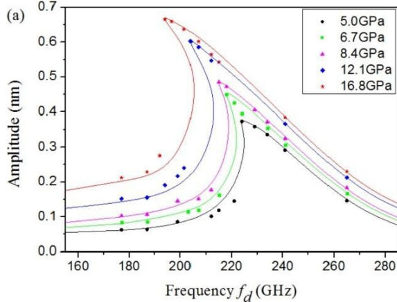
图 31 (a) 锯齿型蜂窝的非线性幅频特性曲线 (b) 扶手椅型非线性幅频特性曲线 (在 5.0GPa、6.7GPa、8.4GPa、12.1GPa 和 16.8GPa 的纵向谐波激励下, 非线性振幅曲线分别为黑色、绿色、紫色、蓝色和红色; 所有仿真的激励频率在 155GHz 到 285GHz 之间。) [140]
