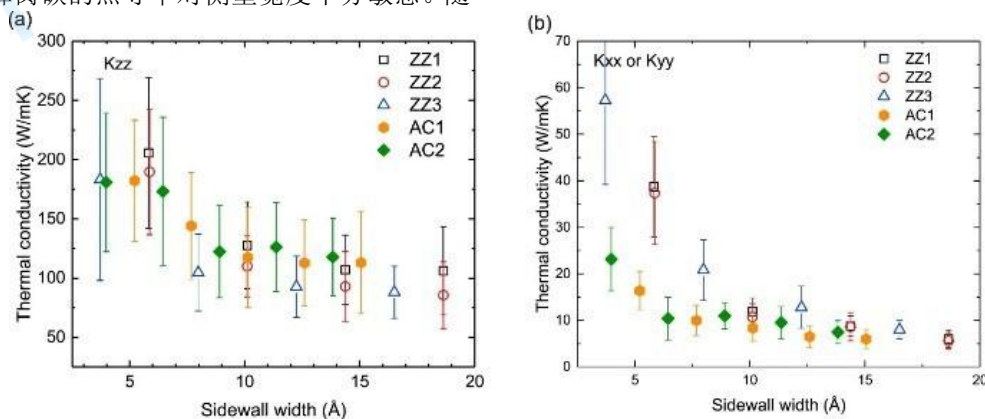
图 23 计算得到的蜂窝碳导热系数随侧壁宽度变化曲线 (a) 沿胞轴方向 (b) 沿扶手椅和锯齿型方向 [106]
