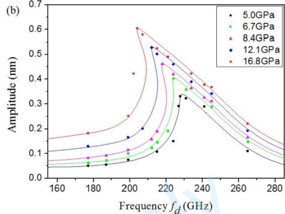
图 31 (a) 锯齿型蜂窝的非线性幅频特性曲线 (b) 扶手椅型非线性幅频特性曲线 (在 5.0GPa、6.7GPa、8.4GPa、12.1GPa 和 16.8GPa 的纵向谐波激励下, 非线性振幅曲线分别为黑色、绿色、紫色、蓝色和红色; 所有仿真的激励频率在 155GHz 到 285GHz 之间。) [140]
