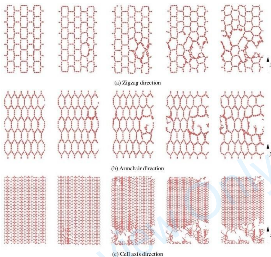
图 14 蜂窝碳失效时的断裂演化过程 (a) 沿锯齿方向拉伸断裂前, CHC 孔为矩形 (b) 沿扶手椅方向拉伸破坏前, CHC 孔为六边形 (c) 沿管轴方向拉伸时 CHC 结构横截面上的断裂演化过程 [81]
