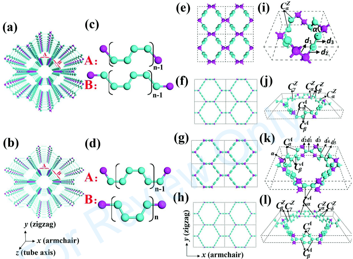
图 6 稳定碳蜂窝的原子结构 (a) Cmc m -CHC-n 形式的结构 (b) Cmmm-CHC-n 形式的结构 (c) Cmc m -CHC-n 形式的重复单元 (d) Cmmm-CHC-n 形式的重复单元 (e-h) 分别为超胞优化后的 Cmc m -CHC-1、Cmc m -CHC-2、Cmmm-CHC-1、Cmmm-CHC-2 俯视结构图 (由紫色的连接原子和蓝色的石墨烯纳米带组成) (i-l) 分别对应于 (e-h) 中原始单元的侧视图 ( d_n' 表示键长, C_{\alpha, \beta, \gamma, \delta}^{Z, A} 表示键角: Z 为之字形方向, A 为扶手椅形方向) [54]
