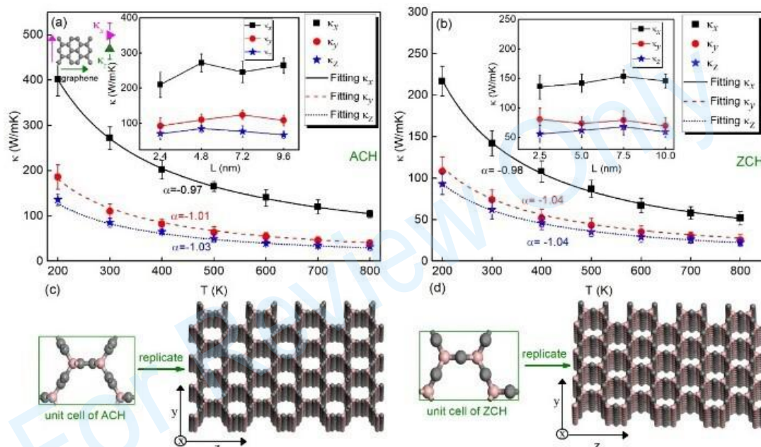
图 24 (a) 扶手椅型蜂窝碳热导率随温度的变化 (b) 锯齿型蜂窝碳热导率随温度的变化 (插图表示晶格尺寸对蜂窝碳热导率的影响) (c) 扶手椅型蜂窝碳的原子结构 (d) 锯齿型蜂窝碳的原子结构 (灰色表示 sp^2 杂化形式的碳原子, 红色表示 sp^3 杂化形式的碳原子) [113]
