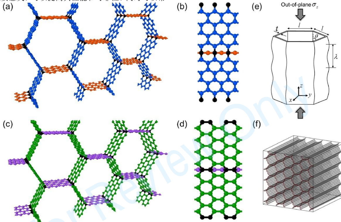
图 21 (a) 和 (c) 分别是扶手椅型和锯齿型蜂窝碳结构。(b) 和 (d) 分别是与 (a)、(c) 所示蜂窝相对应的结处的详细原子构型的放大视图。(e) 沿蜂窝晶格的轴线对蜂窝施加单轴平面外变形。(其中蜂窝晶格的边长为 l , 厚度为 t , 角度为 \theta , 屈曲波长为 \lambda ) (f) 模拟使用的立方周期性超胞。 [53]
