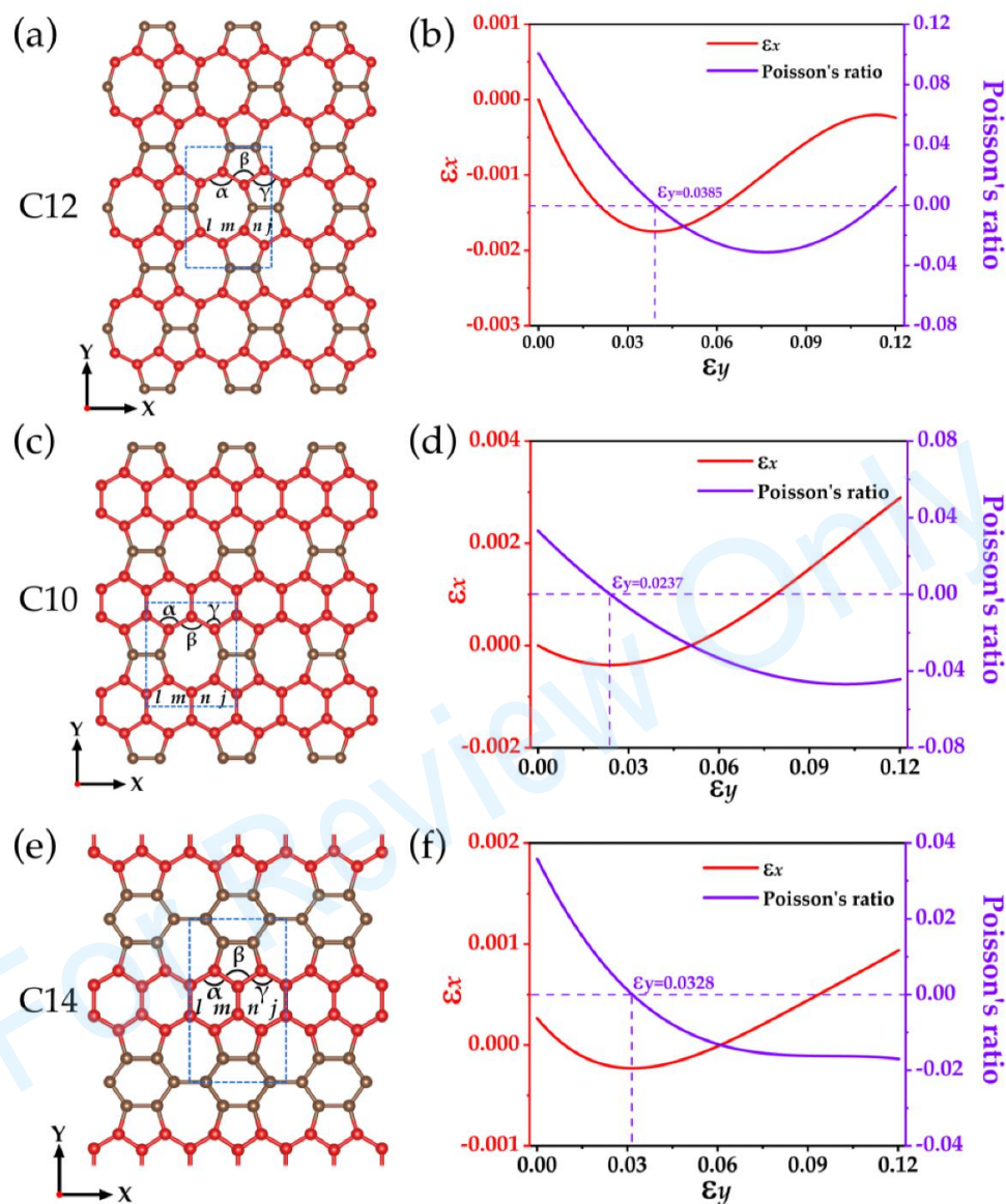
图 20 C10、C12、C14 三种碳结构及其力学响应 (a, c, e) 三种包含锯齿型碳结构被分别标记为 C10、C12、C14。(其中 \alpha, \beta, \gamma 分别表示键角, l, m, n, j 分别表示键长。蓝色矩形表示每种结构的单胞形式, 红色部分则是锯齿型结构) (a, c, e) 三种结构的力学响应分别在 (b, d, f) 中显示 (其中红线表示沿 y 轴单向应变下的响应, 紫线表示沿 y 轴的泊松比变化)
