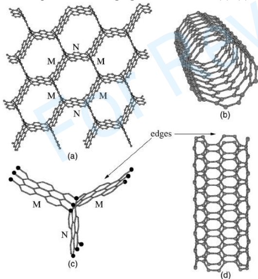
图 3 (a) (3,3) 型的扶手椅形碳泡沫结构 (c) 扶手椅形碳泡沫连接处结构 (b, d) 与其相对应的扶手椅形碳纳米管结构及连接情况 [32]
