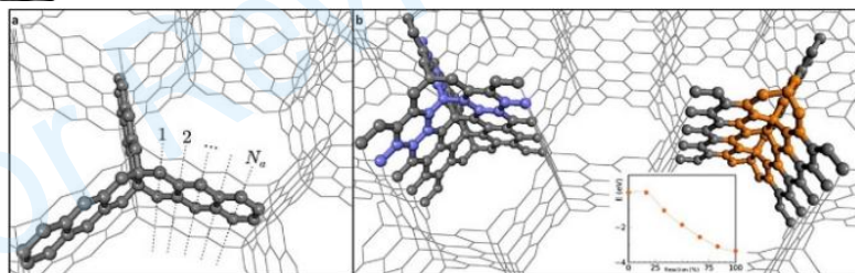
图 5 蜂窝结构 (a) 当 N_a=5 时用球棒法表示的扶手椅型蜂窝晶格 (b) N_z=2 时的锯齿型蜂窝晶格 (紫色部分是原始铰链, 橙色部分是重建铰链, 同时插入了单胞重建过程的能量变化) [51]
