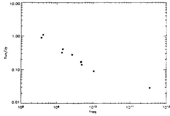
(b) NGC 6137
