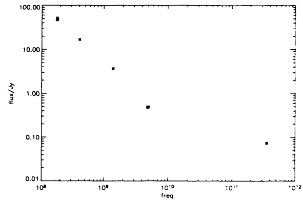
(d) NGC 6166
