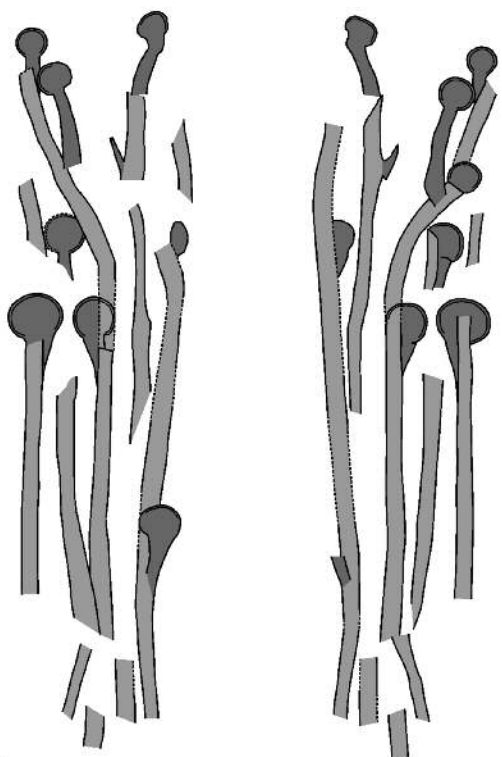
Type 3b: Craswallia haegensis gen. et sp. nov.
