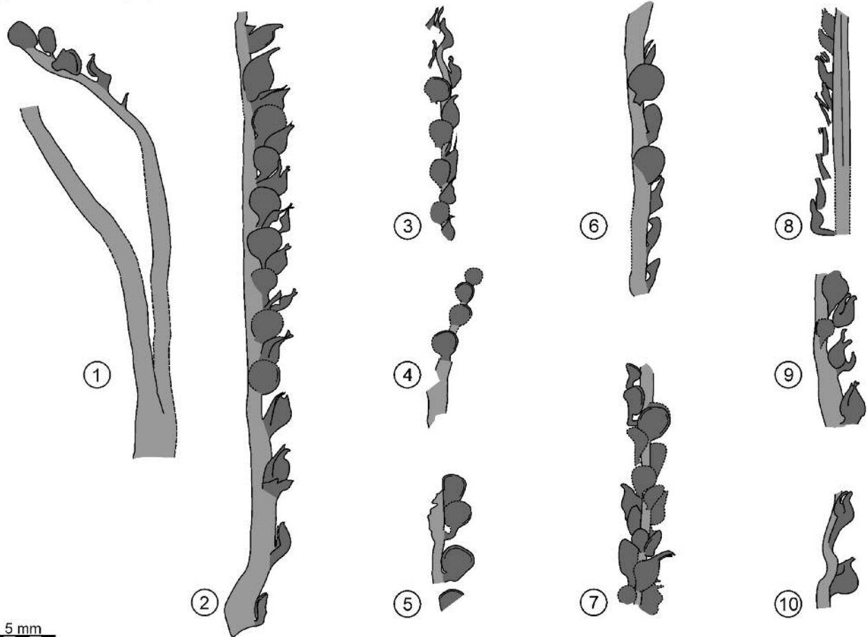
Type 3b: Craswallia haegensis gen. et sp. nov.
