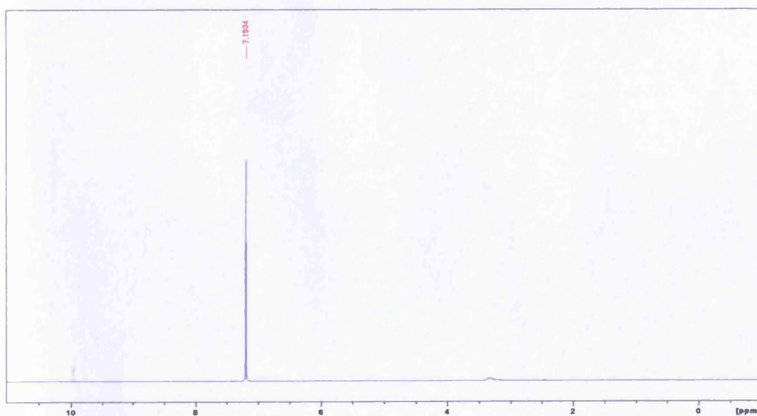
Fig 3.4: ^2\text{H} -NMR of 53
