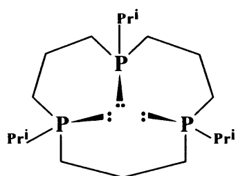
syn-syn
