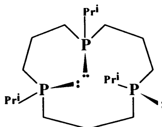
syn-anti
