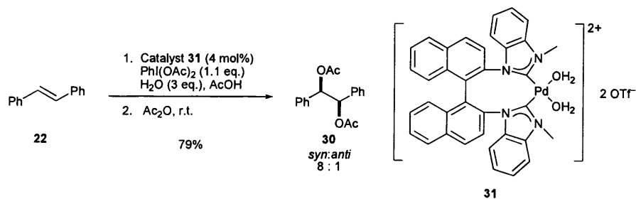
Scheme 1.4
