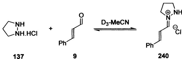
(Scheme 61)
