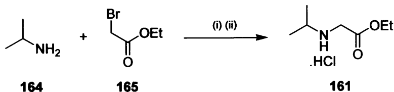
(Scheme 38)
